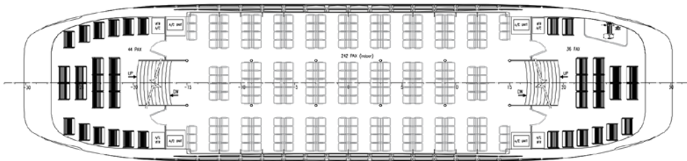
Upper Deck 8150 mm x 19 m B.L.
